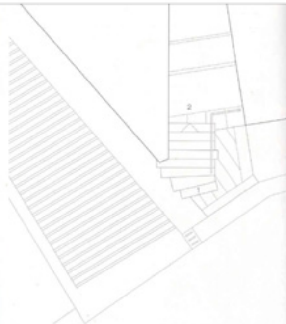
Treppensituation Maßstab 1:100
